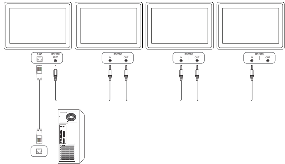
Схема подключения 3
