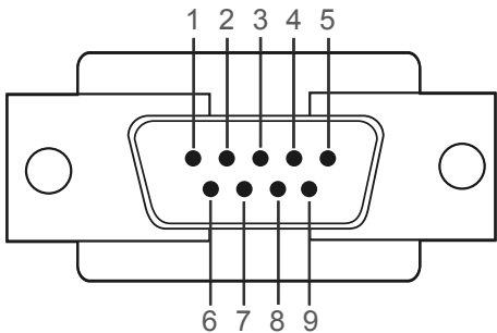
Назначение контактов
