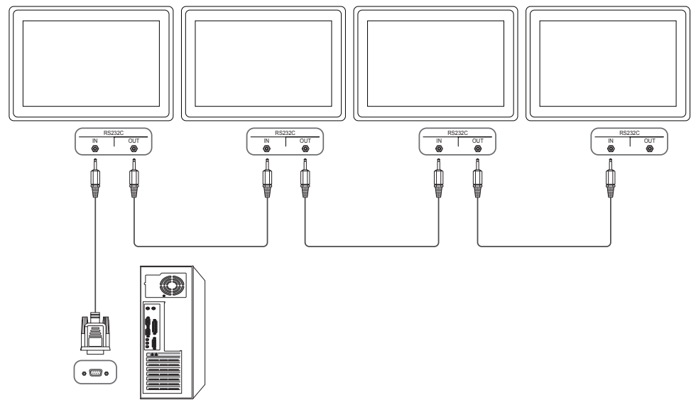
Схема подключения 2
